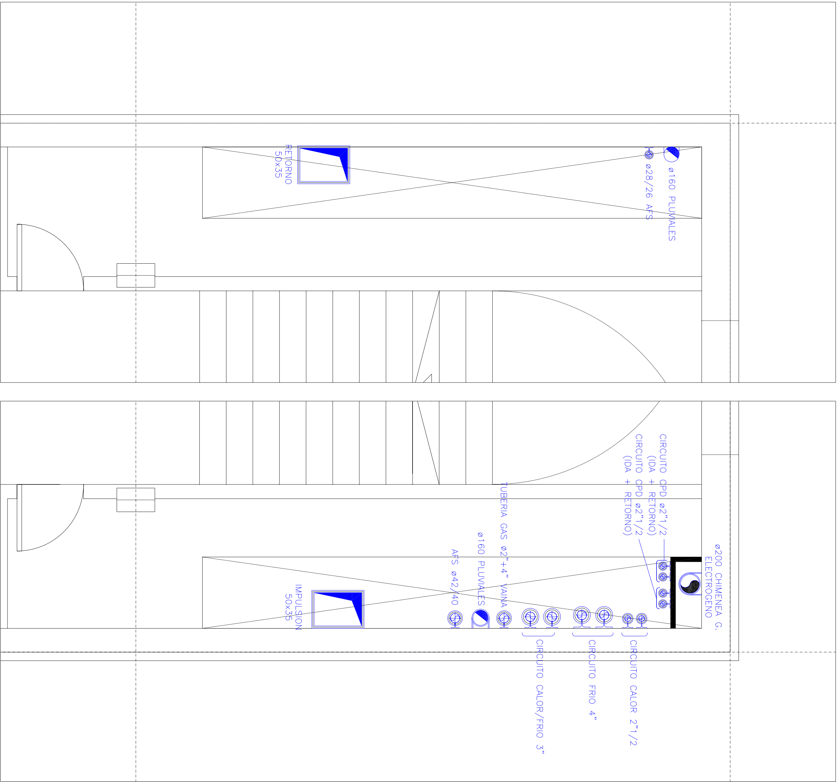
2 PATINILLO 1. PLANTA PRIMERA
