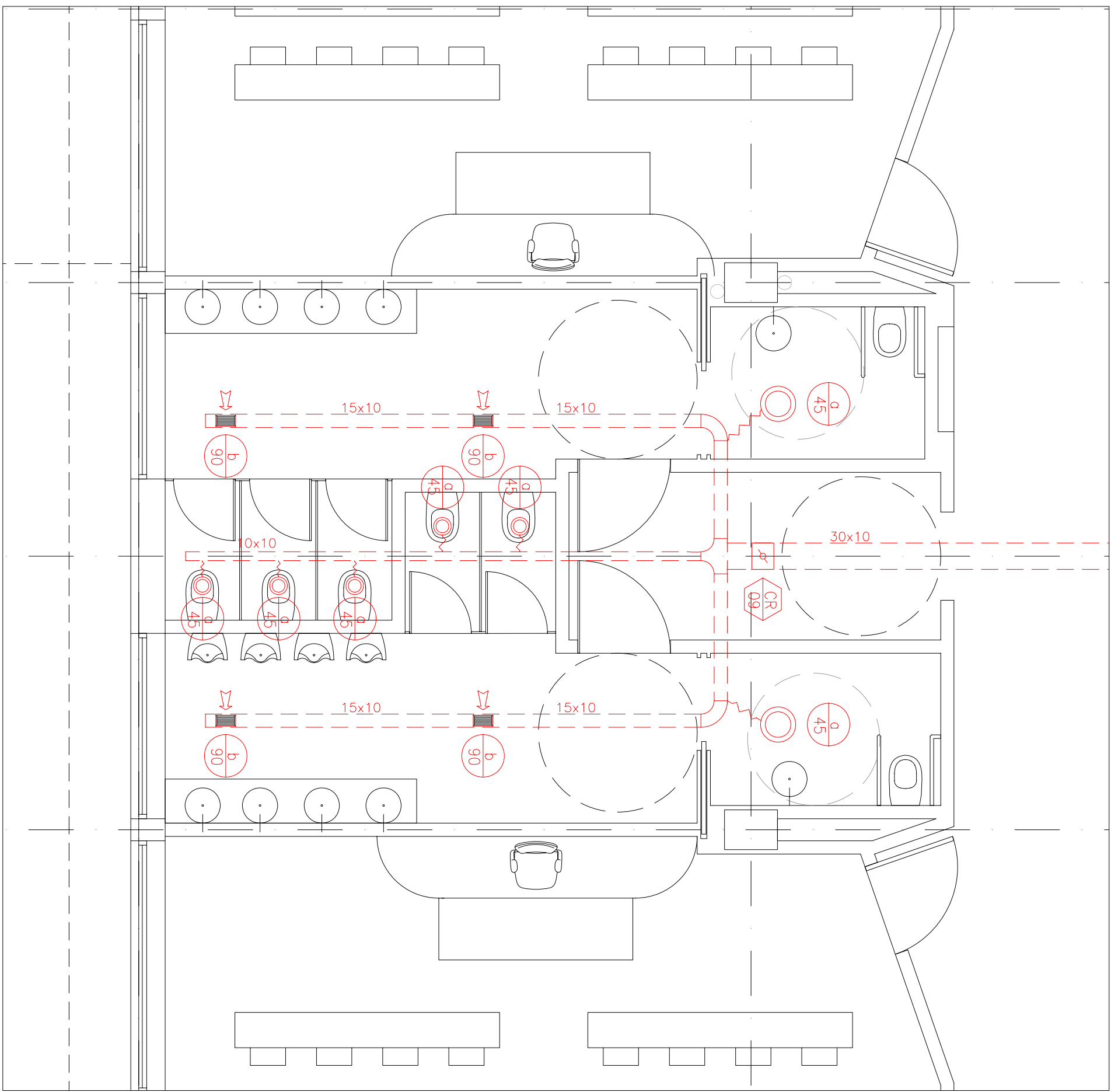
1 PLANTA BAJA. NUCLEO HUMEDO
