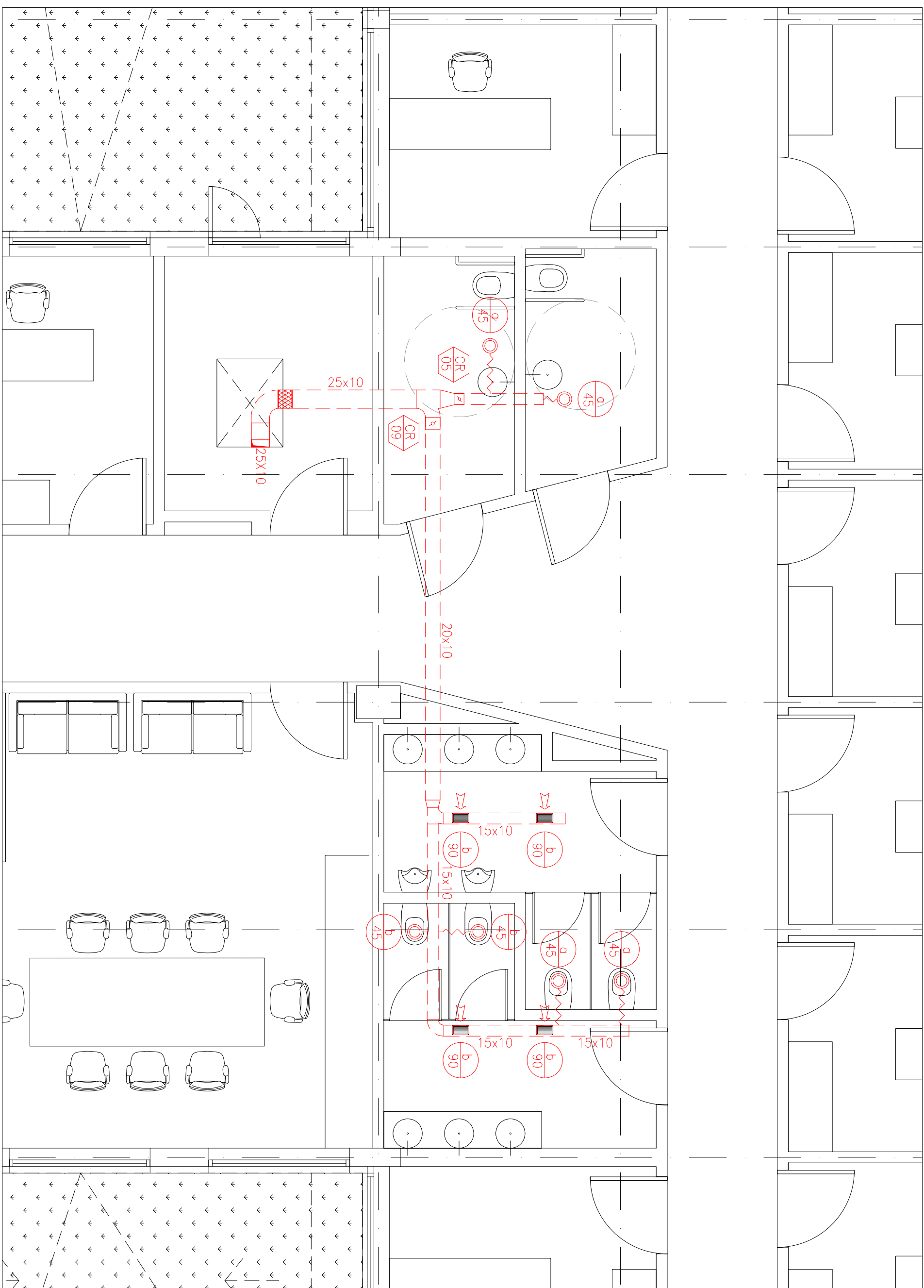
2 PLANTA SEGUNDA. NUCLEO HUMEDO
